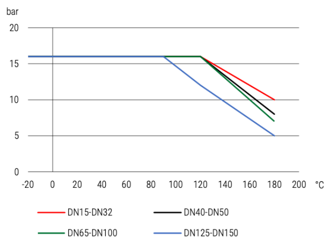
Druck-Temperatur-Diagramm pressure-temperature-diagram
