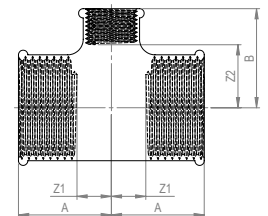
Abzweig vergrößert
