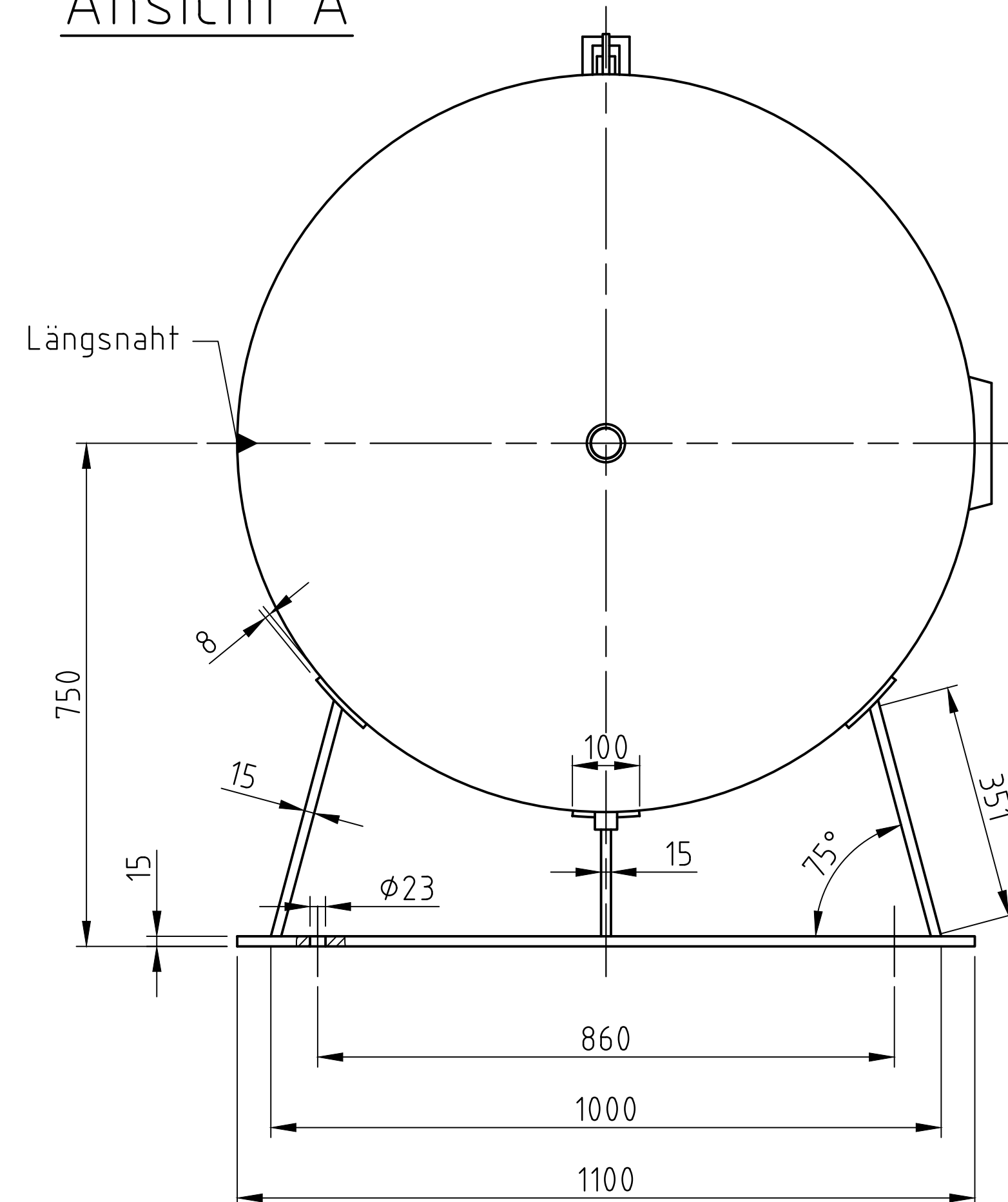
Ansicht A
